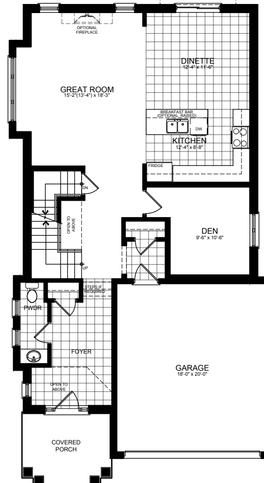
ELEV. A
