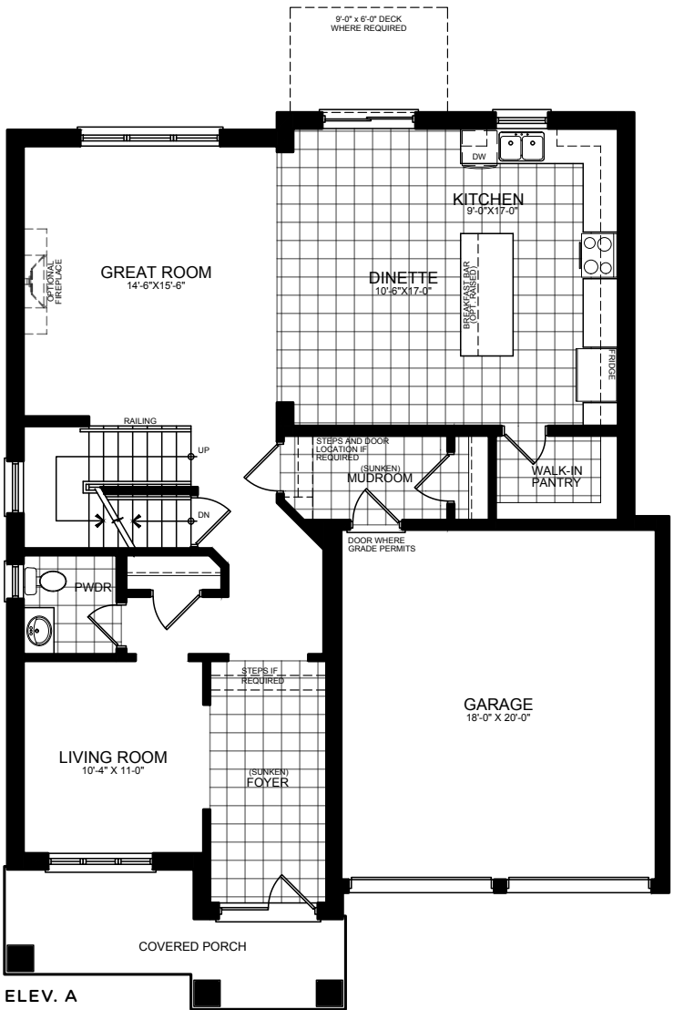
ELEV. A
