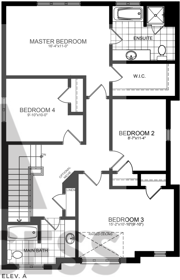
ELEV. A
